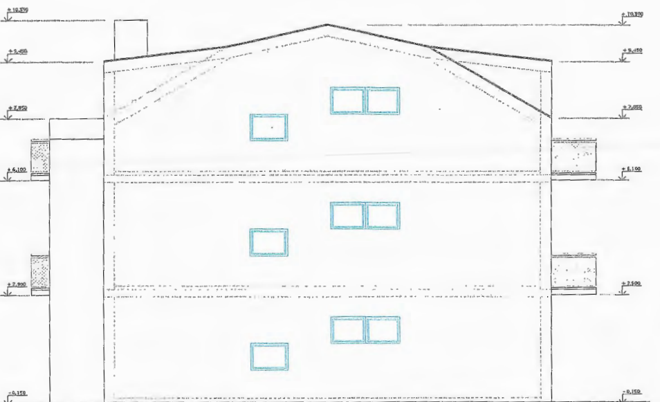
POHLED SEVERNÝ
