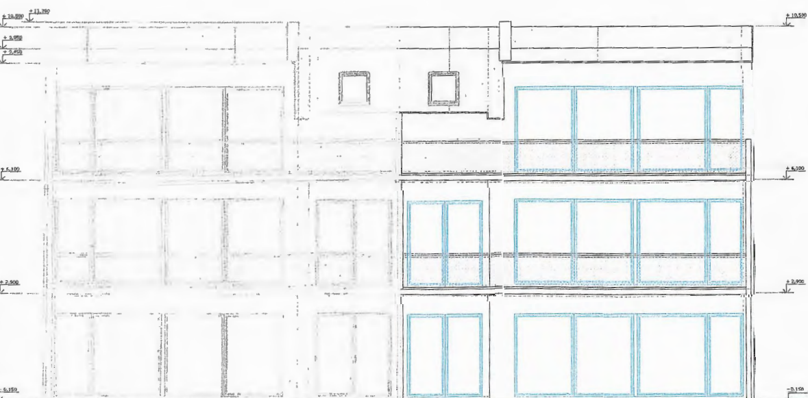
POHLED VÝCHODNÝ
