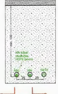
Rez C - C' KOMUNIKÁCIA
