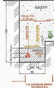
Rez B - B' TERÉN
